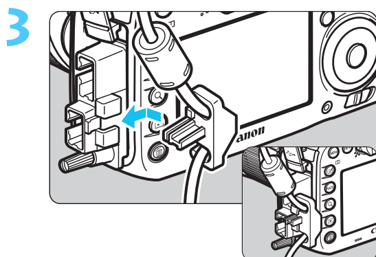
Serre-câbles
