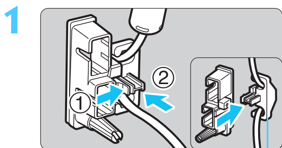
Serre-câbles
