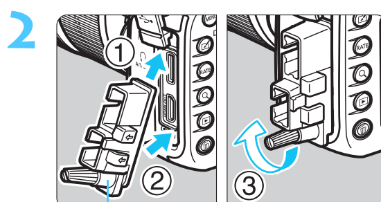
Protecteur de câble
