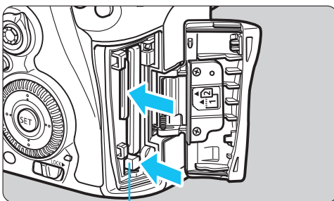
Bouton d'éjection de la carte CF
